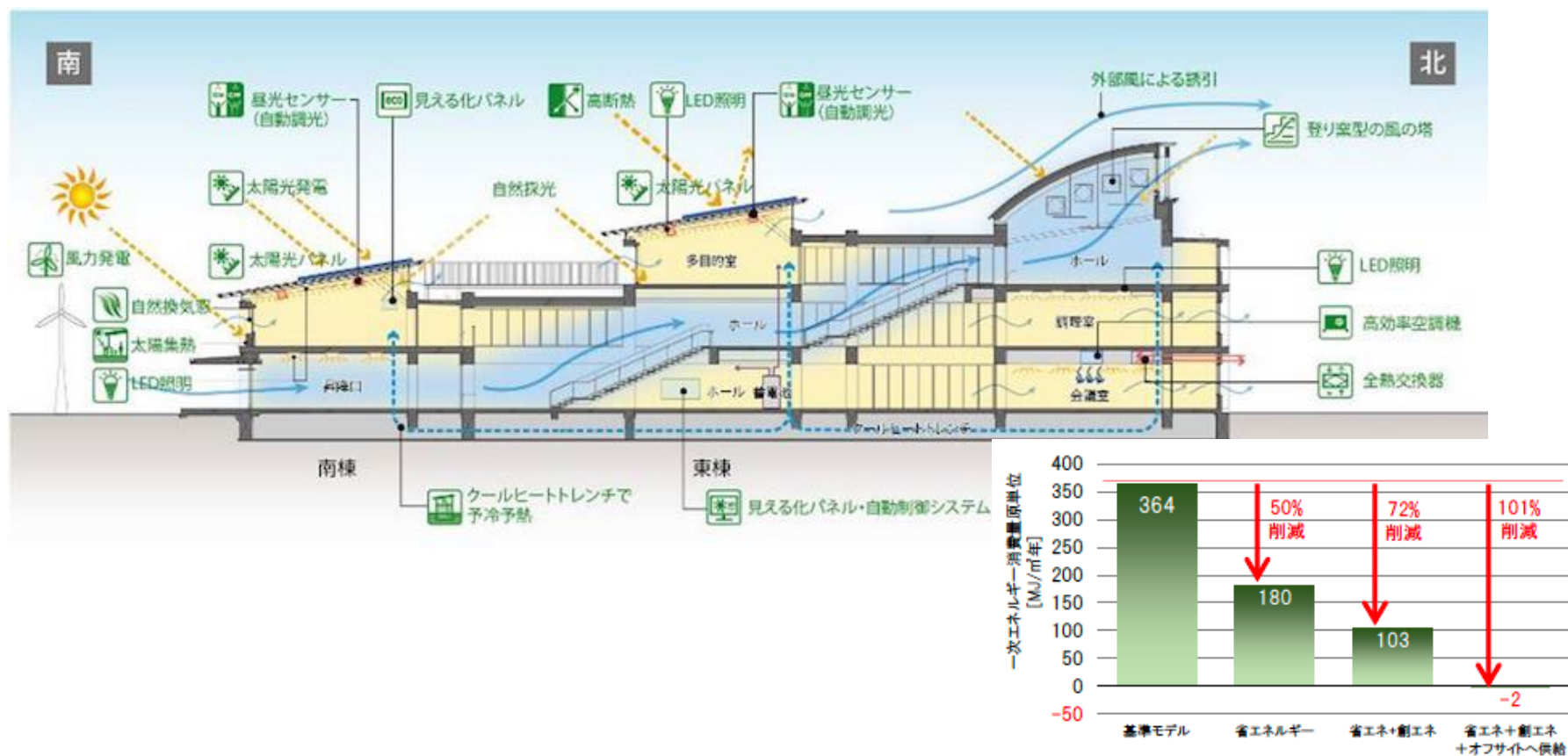
図1 学校の1次エネルギー消費量原単位実績
